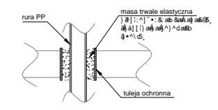
Detal przejścia rury przez przegrody budowlane
